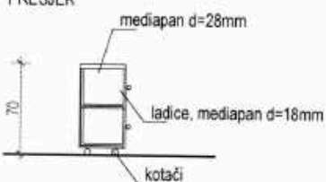
PRESJEK
